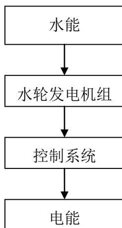
图 3.2-1 工艺流程图
